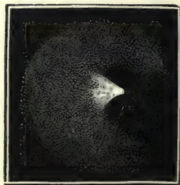
Aug. 29.
